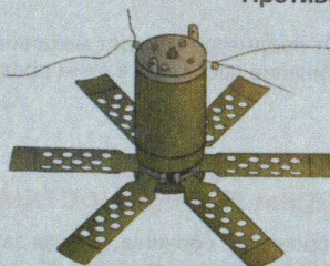
Противопехотная мина ПОМ-2
