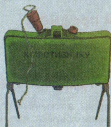
Противопехотная мина МОН-50
